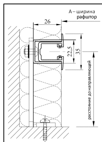
VL7 — Скрытая направляющая специальным коробом ZP
